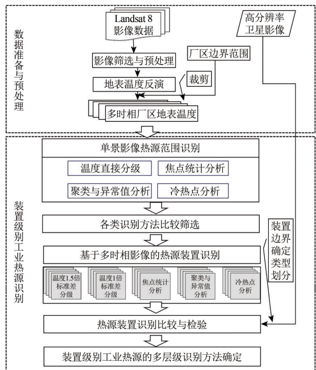
图 2 基于 Landsat 8 的装置级别工业热源的多层级识别技术路线
