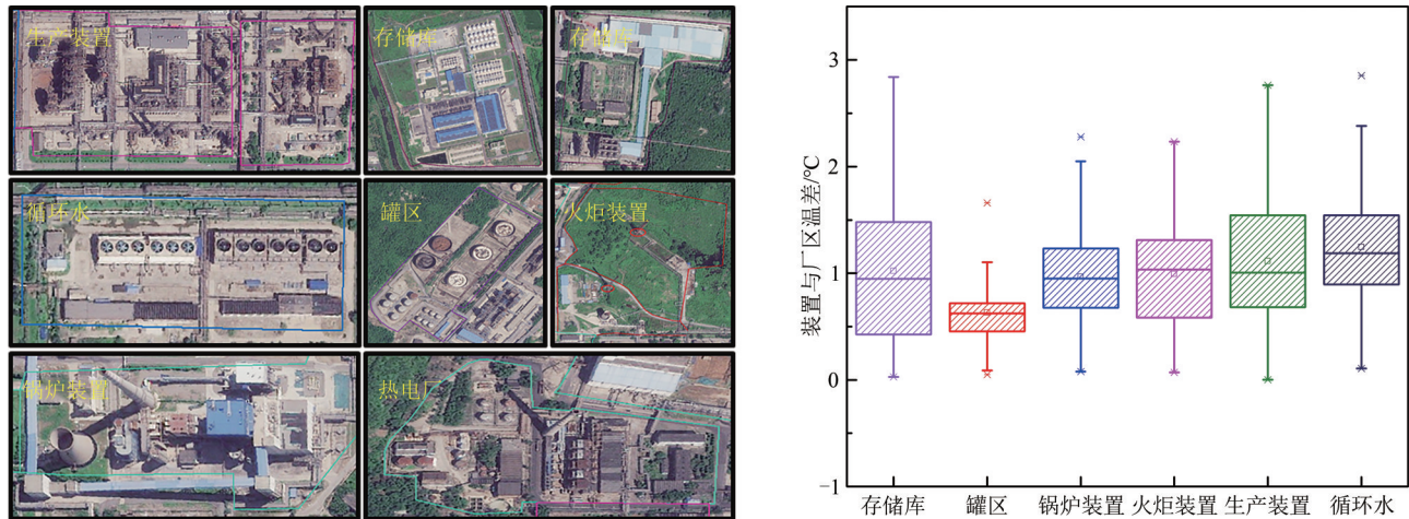
图 10 热源装置典型影像特征及温度特征
