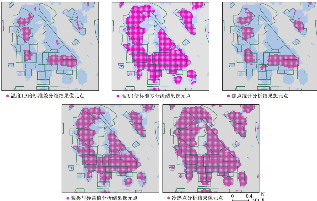
图9 各方法识别的像元落入参考范围的情况(以D生产区为例;绿色边界:参考范围;浅蓝色阴影:冷热点分析识别结果范围)
